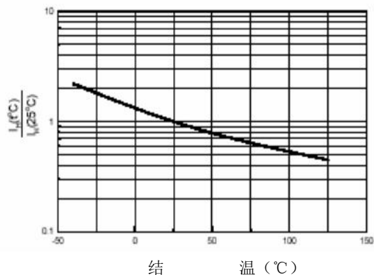
图七、典型维持电流
