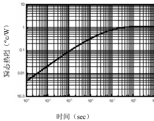
图四、热响应
