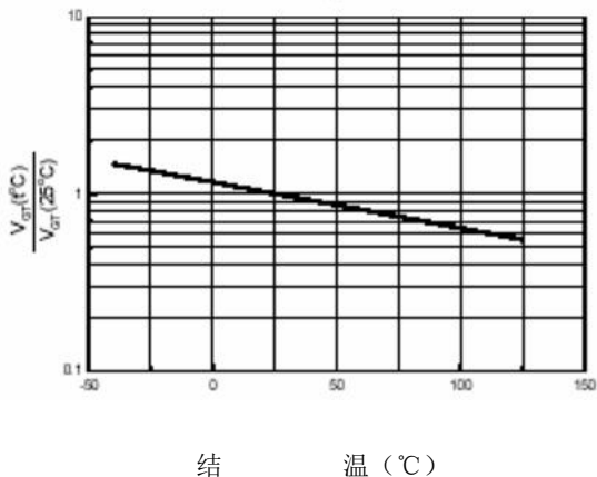
图五、典型门极触发电压----结温
