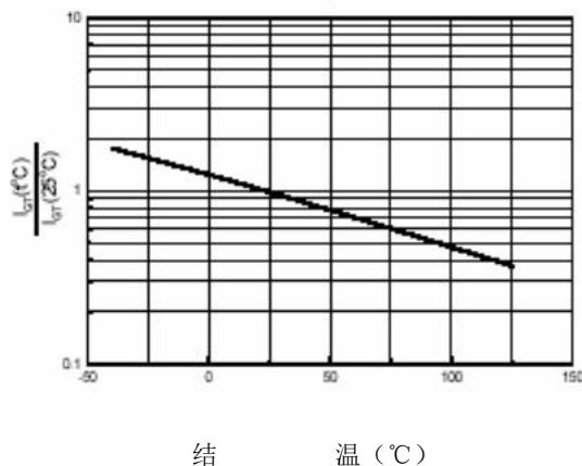
图六、典型门极触发电流----结温
