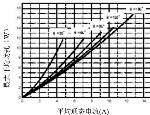
图八、功耗
